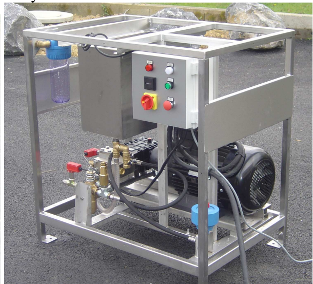
Nettoyeur 500Bar 16L/Min 25cv fixe
